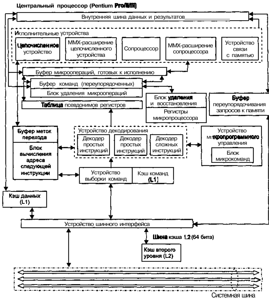
Рис. 2.3. Структурная схема процессора семейства P6 (Pentium Pro/11/III)
