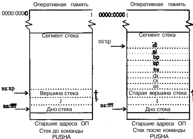
Рис. 7.6. Принцип работы команды PUSH
