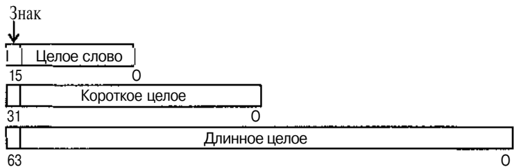
Рис. 17.5. Форматы целых чисел сопроцессора
