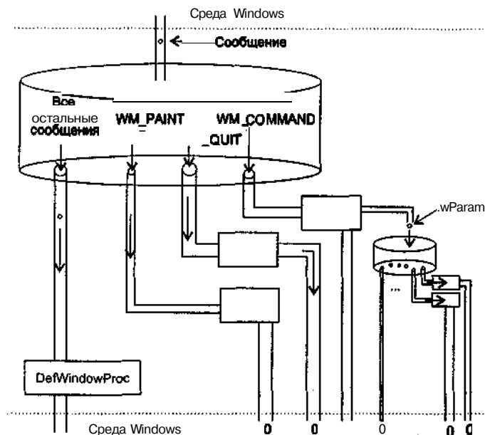
Рис. 16.1. Абстрактное представление структуры оконной функции Windows
