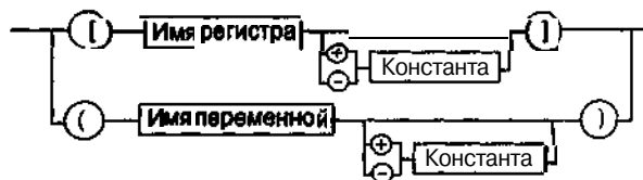
Рис. 13.1. Синтаксис адресного выражения в операторе обращения к полю структуры
