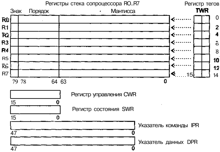
Рис. 17.1. Программная модель сопроцессора
