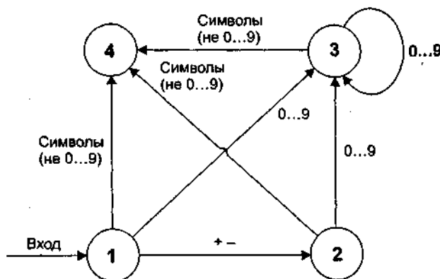
Рис. 11.1. Конечный автомат для десятичного числа со знаком
