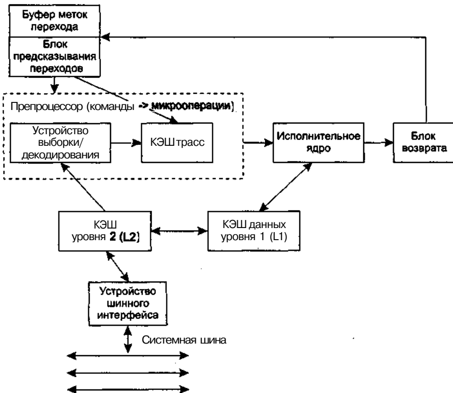
Рис. 2.4. Структурная схема процессора Pentium IV
