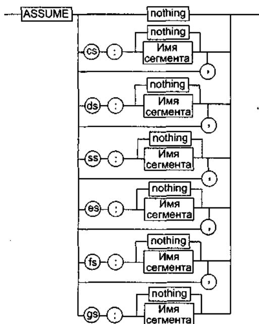
Рис. 5.15. Директива ASSUME
