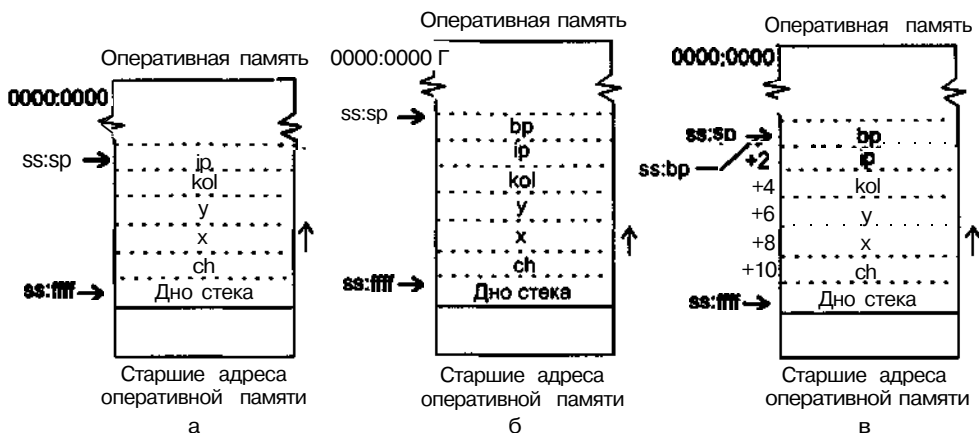
Рис. 15.3. Изменение содержимого стека при передаче управления в связке C-ассемблер
